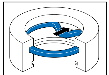
1A. Einbau mit Montagezange | Montaj pensesi ile montaj | Instalacja za pomocą szczypiec | Установка с помощью монтажного инструмента
