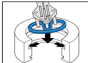
1A. Einbau mit Montagezange | Montaj pensesi ile montaj | Instalacja za pomocą szczypiec | Установка с помощью монтажного инструмента
