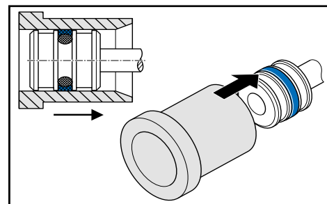
Instalacja za pomocą taśmy montażowej i tulei kalibracyjnej | Установка с помощью монтажной ленты и калибровочной втулки
